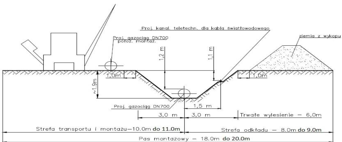
Rys.4. Poglądowy schemat zagospodarowania pasa montażowego - tereny leśne
