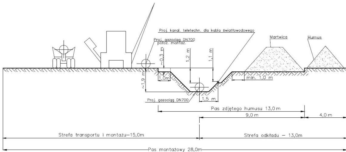
Rys. 3. Poglądowy schemat zagospodarowania pasa montażowego w trakcie budowy - tereny rolne
